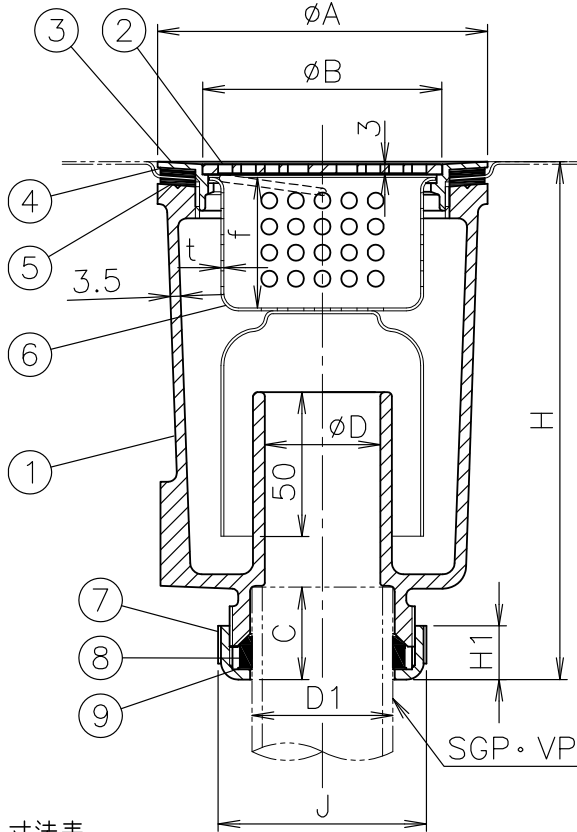
寸法表
