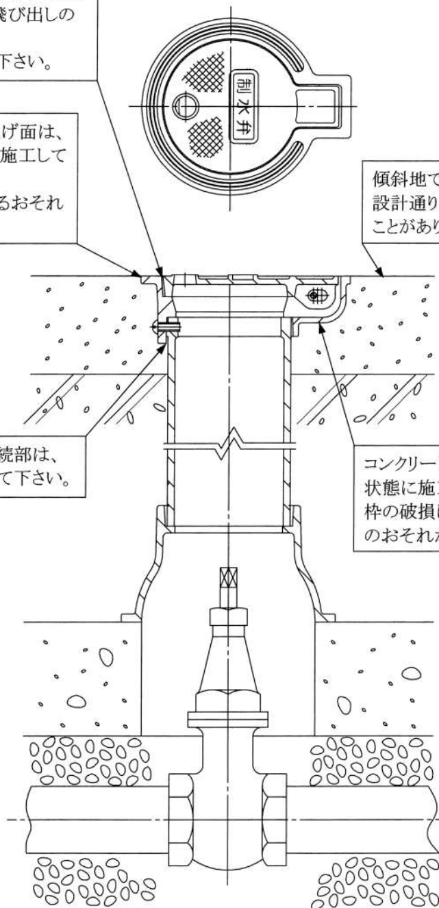
施工例:B5
