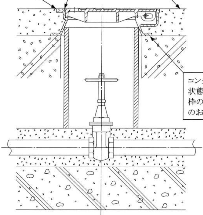
施工例:B-1
