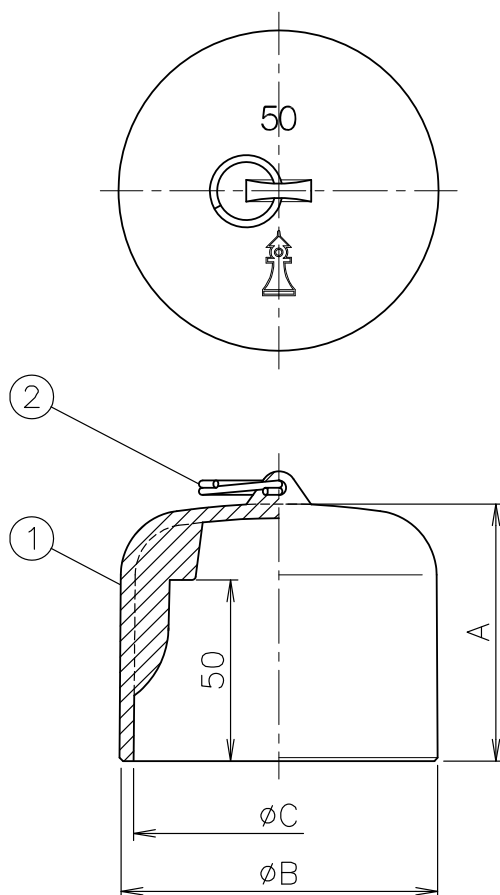
寸法表 単位:mm
