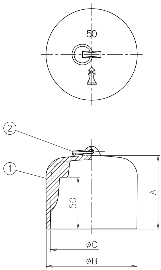
寸法表 単位:mm
