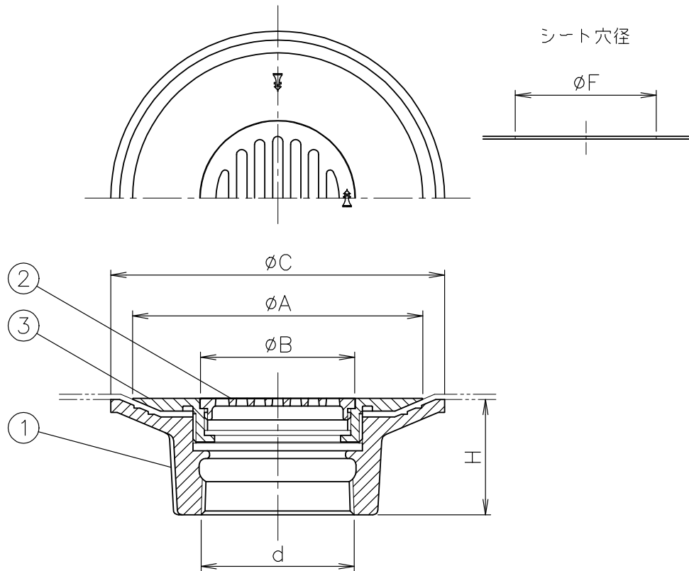
寸法表
