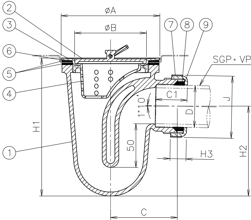
寸法表
